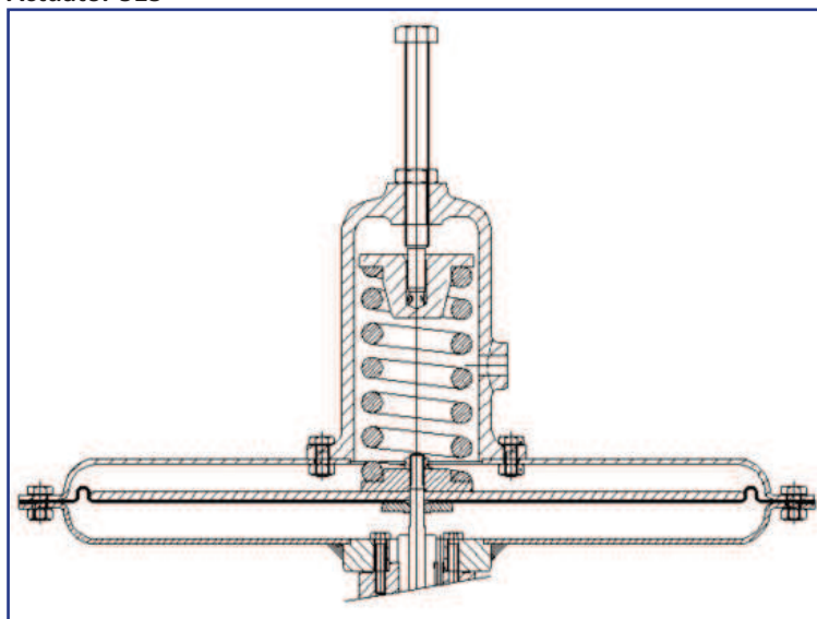
Actuator 515
