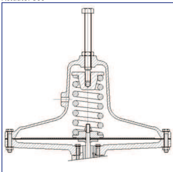
Actuator 360
